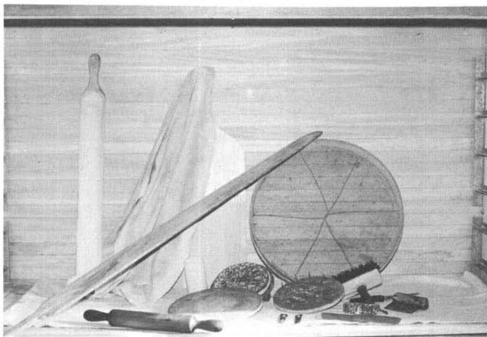
Alguno de los utensilios utilizados en panadería: caña, palín, pala —sin mango—, tela, criba o cernedora, bote para medir la sal, rodillo de masa, tabla de madera para coger pan de flama, pica, cepillo de dar agua, cuchillo, rascas, rasquetas, sellos para marcar el pan y cuchillas.
