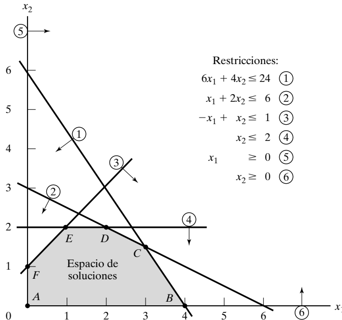
FIGURA 2.1 Espacio factible del modelo de Reddy Mikks
