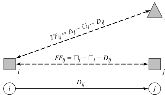
FIGURA 6.58 Cálculo de las holguras totales y libres
